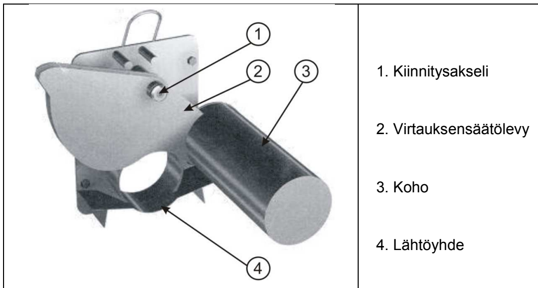
Kuva 10. Virtauksensäätkäimen osat.
